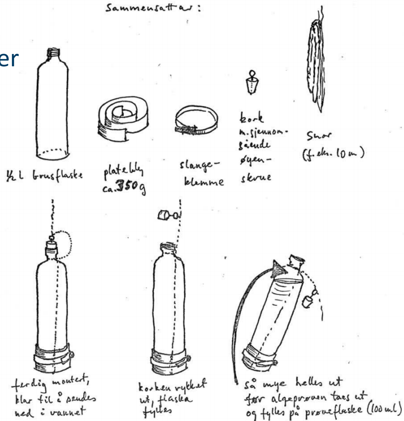
Figur 1 Enkel vannhenter ("Flaskevannhenter")
