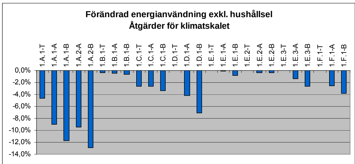
Figur 4.17 Förändrad energianvändning vid åtgärder för klimatskalet
