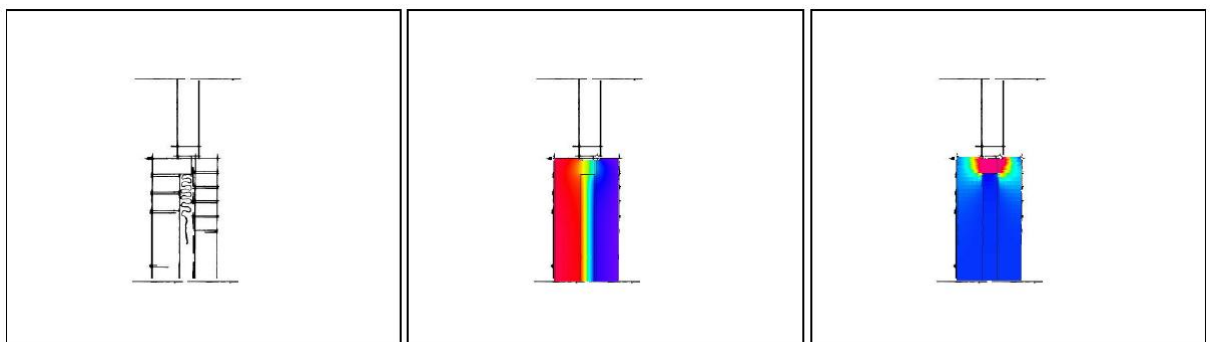
Figur 4.16 Anslutning balkong ovan avväxlingsbalk i lättbetong t v; detaljritning som beskriver köldbryggan, i mitten; temperaturfördelning genom anslutningen, t h effektförlust för anslutningen
