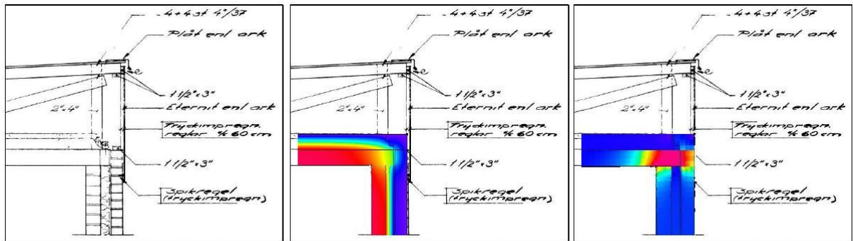
Figur 4.9 Anslutning takbjälklag – yttervägg t v; detaljritning som beskriver köldbryggan, i mitten; temperaturfördelning genom anslutningen, t h effektförlust för anslutningen
