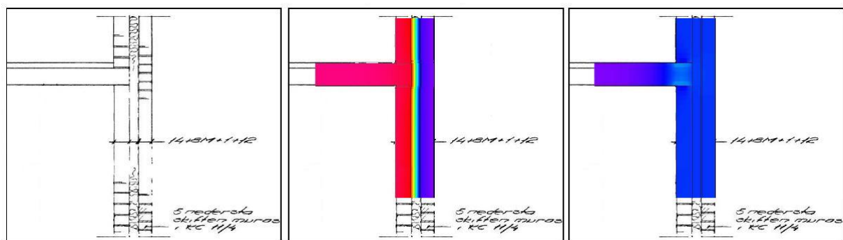
Figur 4.10 Anslutning mellanbjälklag – yttervägg t v; detaljritning som beskriver köldbryggan, i mitten; temperaturfördelning genom anslutningen, t h effektförlust för anslutningen
