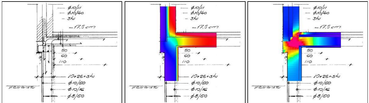
Figur 4.15 Anslutning balkong ovan avväxlingsbalk i lättbetong t v; detaljritning som beskriver köldbryggan, i mitten; temperaturfördelning genom anslutningen, t h effektförlust för anslutningen
