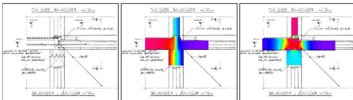
Figur 4.12 Anslutning balkong ovan avväxlingsbalk i lättbetong t v; detaljritning som beskriver koldbryggan, i mitten; temperaturfördelning genom anslutningen, t h effektförlust för anslutningen
