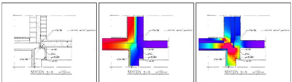
Figur 4.14 Anslutning balkong ovan avväxlingsbalk i lättbetong t v; detaljritning som beskriver köldbryggan, i mitten; temperaturfördelning genom anslutningen, t h effektförlust för anslutningen
