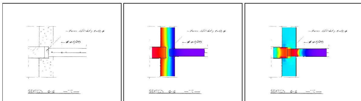
Figur 4.11 Anslutning bärande vägg – balkongflagga t v; detaljritning som beskriver koldbryggan, i mitten; temperaturfördelning genom anslutningen, t h effektförlust för anslutningen
