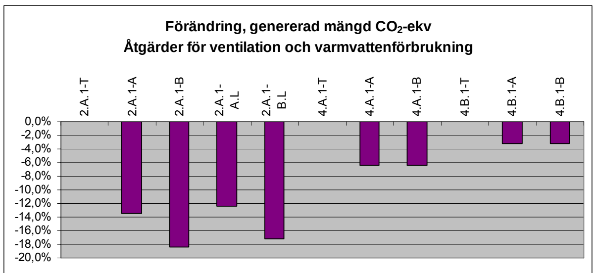
Figur 4.21 Förändring genererad mängd koldioxidekvivalenter vid installation av FTX samt åtgärder för att minska varmvattenförbrukningen
