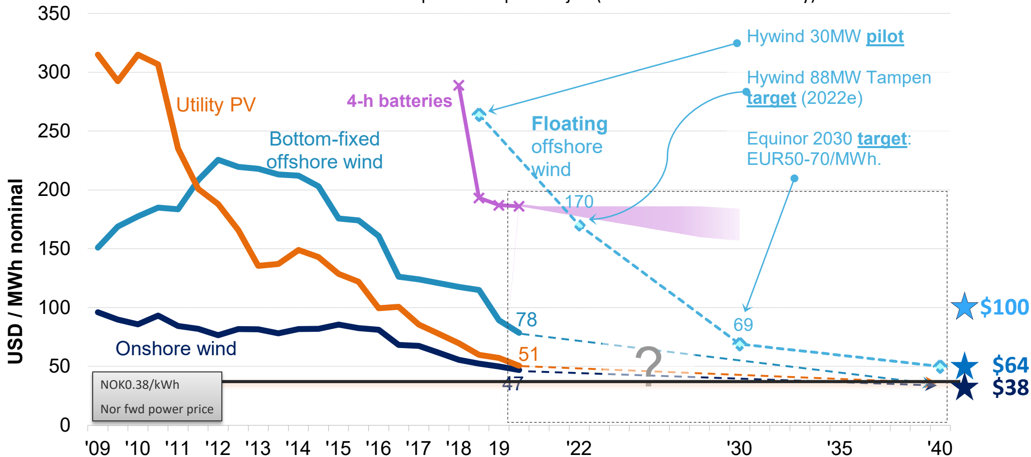
Totale levetidskostnader delt på levetidsproduksjon (Levelized Cost of Electricity)
