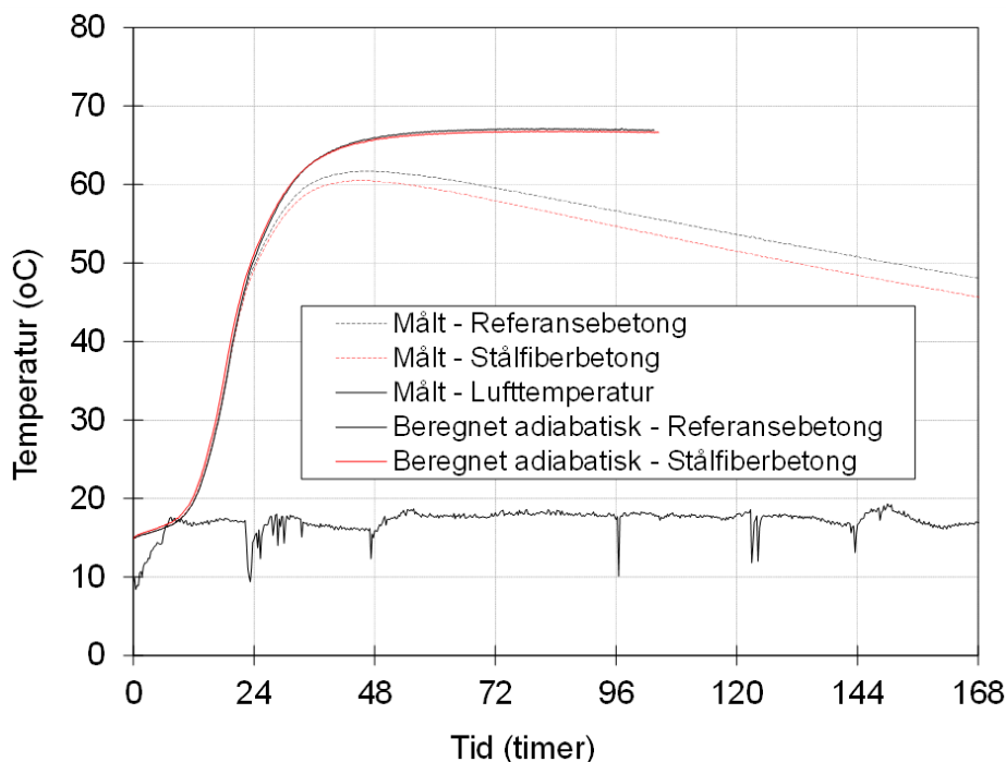
Figur 7 Herdekasseforsøk – målt temperatur i de to herdekassene samt i luft, og beregnet adiabatisk temperaturforløp
