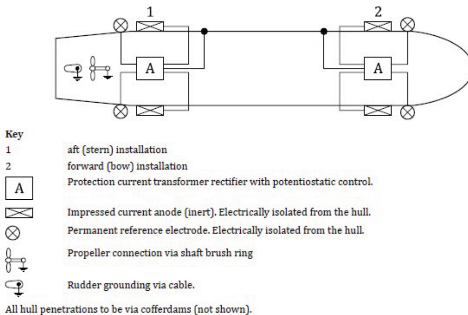
Figur 8. Skjematisk oversikt over anodeplassering for påtrykt strømanlegg på skipsskrog basert på 2 soner (fra ISO 20313)
