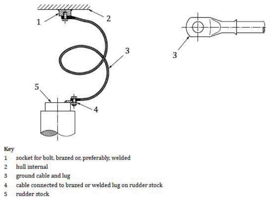
Figur 10. Elektrisk kontinuitet for rørstamme (fra ISO 20313)
