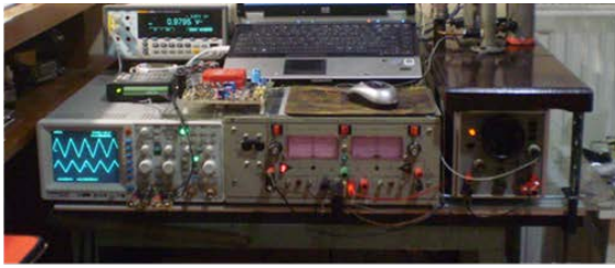
Stand pentru determinarea inovativa a rezistentei de contact interfacial (ICR), realizata in cadrul proiectului
