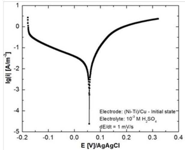
Curbe liniare de polarizare (Tafel pante) pe electrozi (Ni-Ti)/Cu in H 2 SO 4 10 -3 M + 0.1 ppm F- la temperatura ambianta si la o viteza de scanare de 1mV/s.
