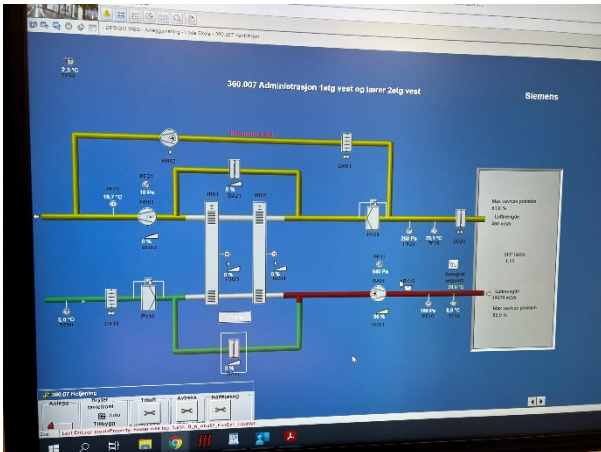
Fig. 2 Oversikt over ventilasjonsaggregatet under test p&aring; Lade skole.
