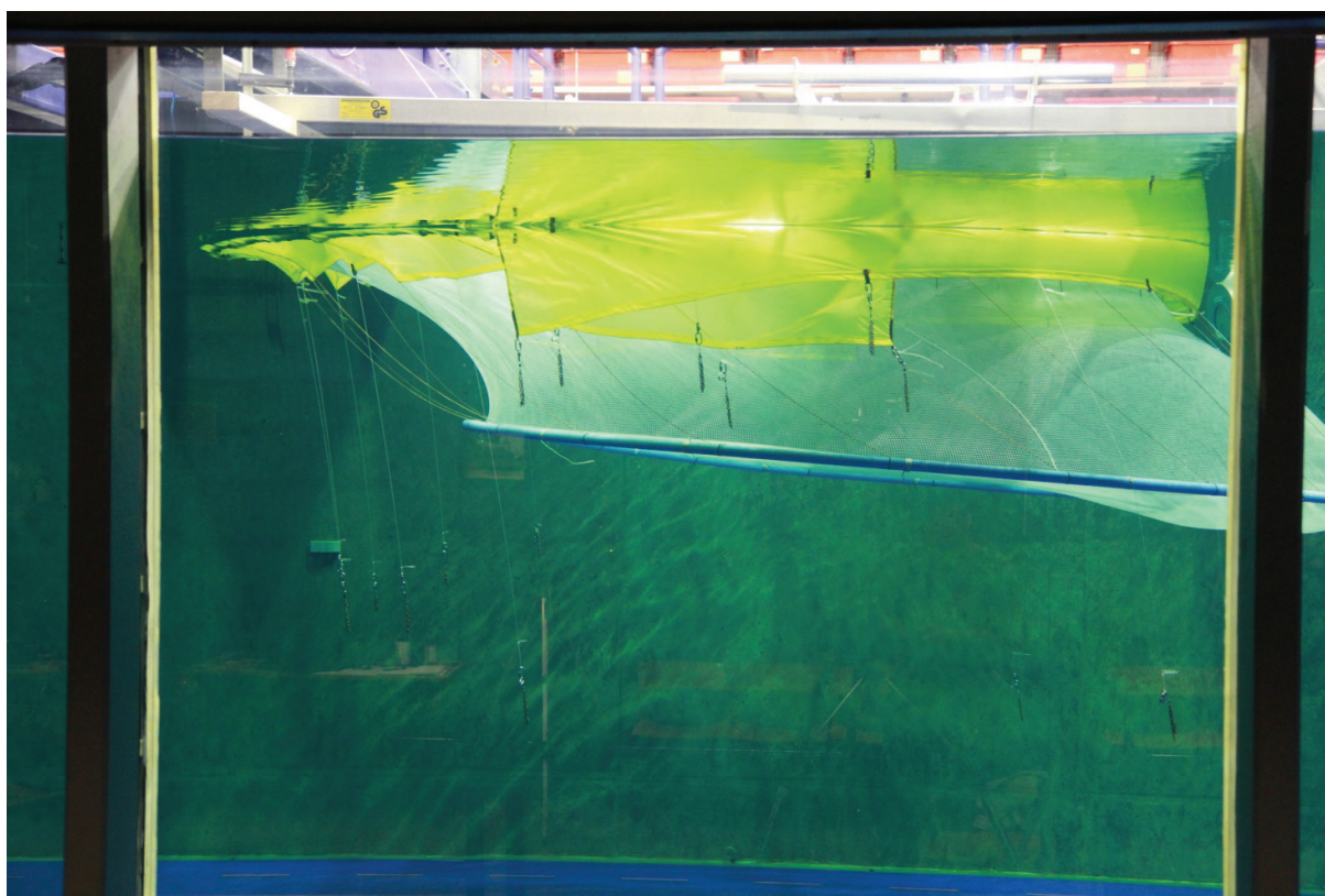
Fig. 4.2.4. Merd med 363 mm skjørt montert med overlapp i motstrøms retning ved 20 \text{ cm s}^{-1} strøm i tanken. Ved denne strømhastigheten ble det tydelig at halvdelen av skjørtet på fremsiden av merden i forhold til strømretningen la seg flat oppunder bunnringkjettingene og nota og halvdelen på baksiden blåste seg opp som et seil.
