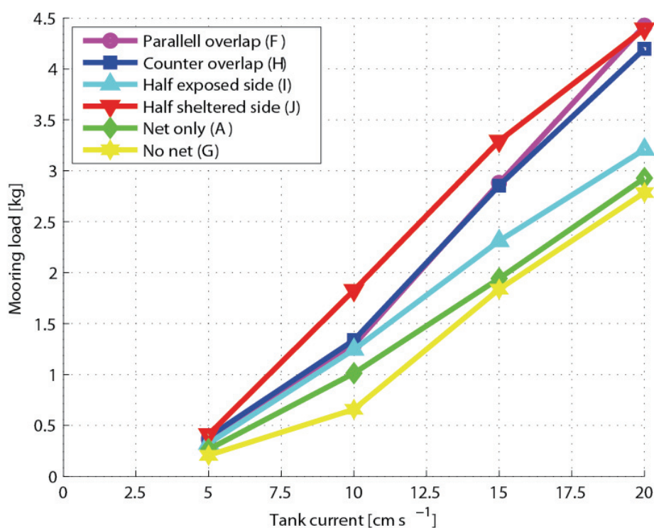
Fig. 4.2.5. Total fortøyningskraft ved ulike strømhastigheter for 363 mm skjørt med 26 x 36 g enkeltlodd. Bokstaven bak hver linje i grafen korresponderer til bokstavene i Fig. 4.2.3.
