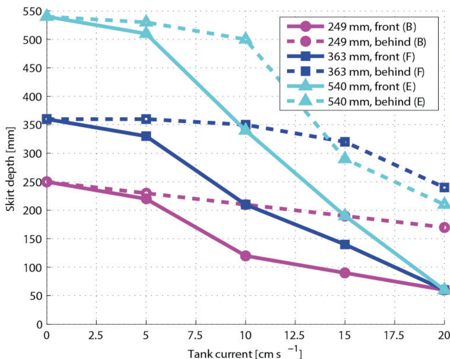
Fig. 4.1.2. Avstand fra underkant av skjørtet til vannoverflaten på fremsiden og baksiden av merden for de tre skjørtene med dybde på henholdsvis 249, 363 og 540 mm. Bokstaven bak hver linje i grafen korresponderer til bokstavene i Fig. 4.1.1.
