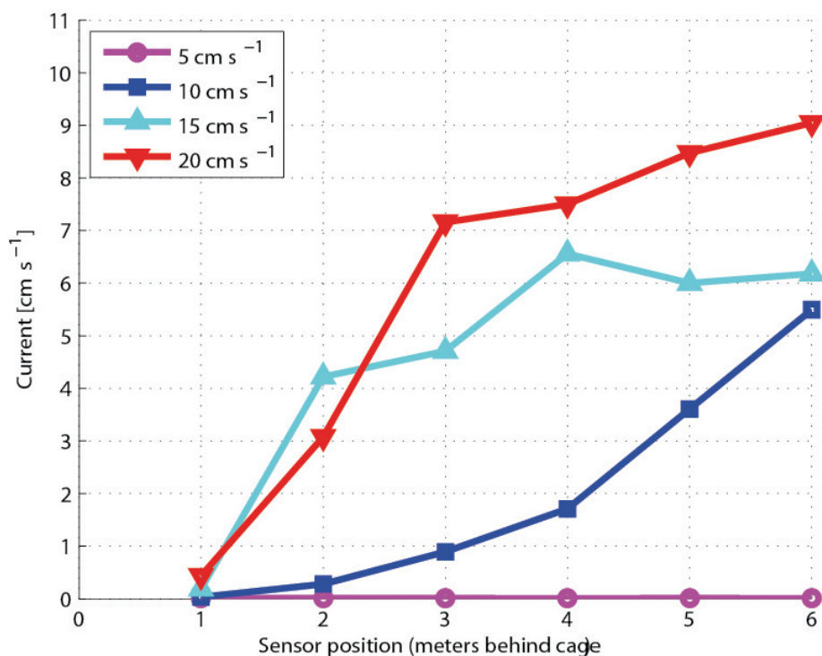
Fig. 4.4.2. Gjennomsnittet av målinger gjort med propellmåler i posisjon P6-P11 med 1 meters mellomrom nedstrøms retning bak merden for merd med 540 mm skjørt loddet med 26 enkeltlodd på 36 g.
