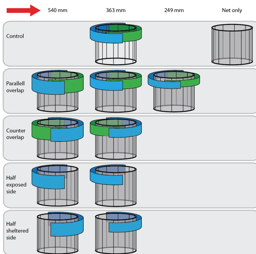
Fig. 3.4.1 Ulike skjørtkonfigurasjoner som ble testet. Alle skjørtkonfigurasjonene ble kjørt med strømhastigheter 5, 10, 15 og 20 cm s -1 i tanken. Den røde pilen viser strømrretningen i tanken.
