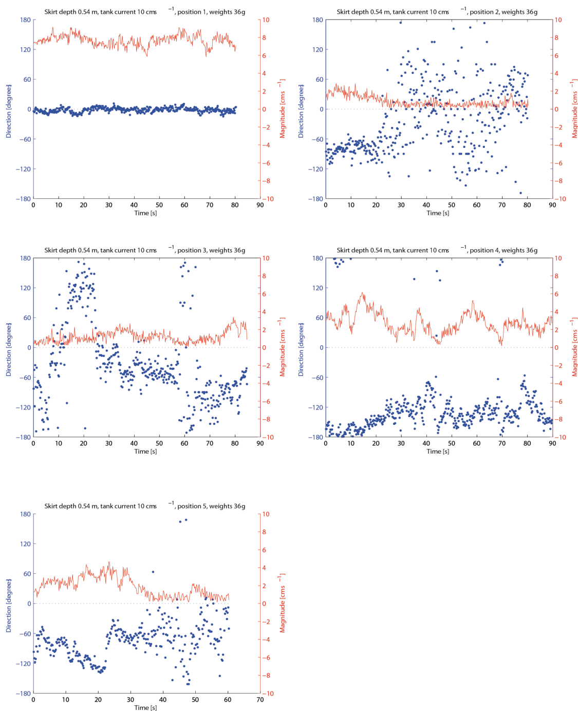
Fig. 4.3.1. Strømfart og retning vist som tidsplott for hver posisjon (P1 – P5) for skjørt med dybde på 540 mm og strømhastighet langs tanken på 10 cms -1 . Strømfart er angitt på y-aksen til høyre, mens retningen er angitt på y-aksen til venstre.
