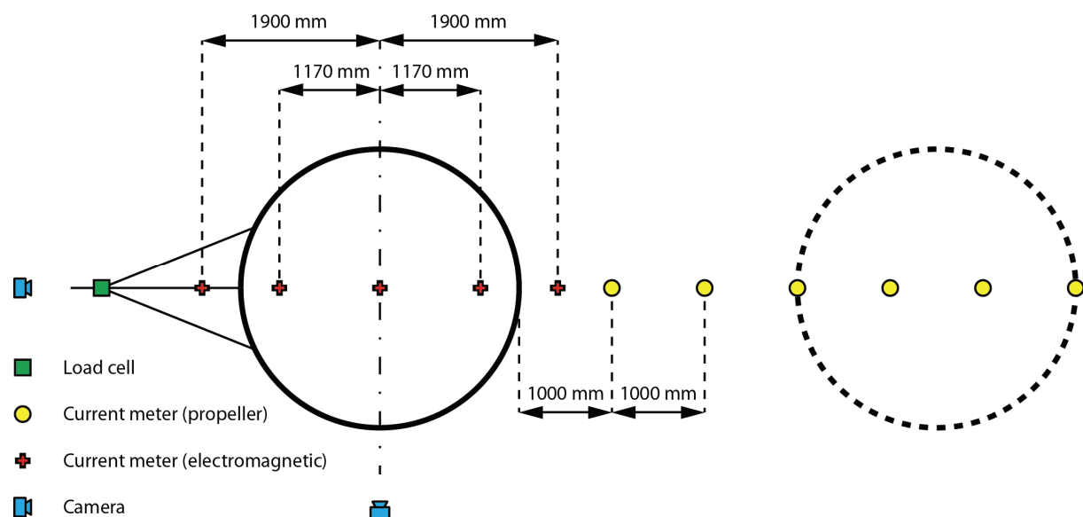
Fig. 3.3.1. Plassering av måleutstyr og kameraer i flumetanken. Propellmåleren måler strøm bak merden for å undersøke hvor sterk strøm en eventuell neste merd nedstrøms opplever som følge av å ligge i skyggen av den foran.
