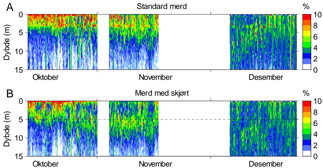
Figur 3.1: Ekkoloddplott for A) standardmerd og B) tilsvarende merd utstyrt med skjørt ned til 5 m (stiplet linje) for lokalitet Saltkjelen, høst 2013. Fargekoden gir et estimat på prosentandel fisk innefor 0,5 m. Svingerne til ekkoloddet stod på mer enn 15 m dyp.
