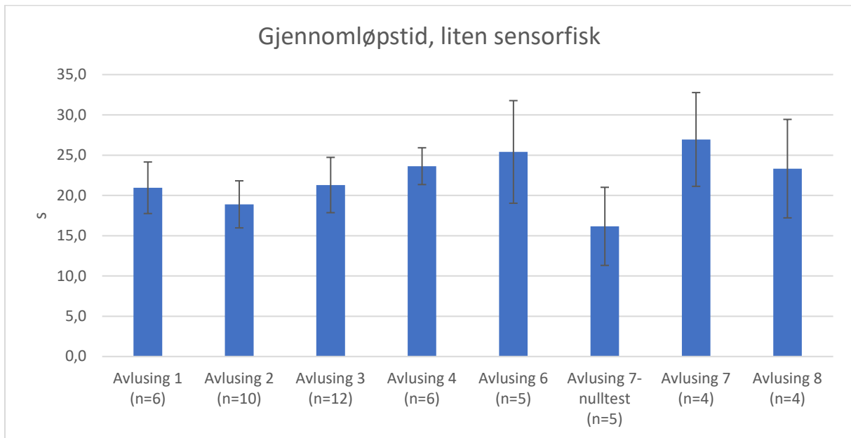
Figur 22 – Pumpetider for liten sensorfisk for Avlusing 1 - 8. Middelerverdi \pm SD. "Nulltest" er gjennomløpstid for sensorfiskene når enhetene for avlusing ikke var innkoblede.
