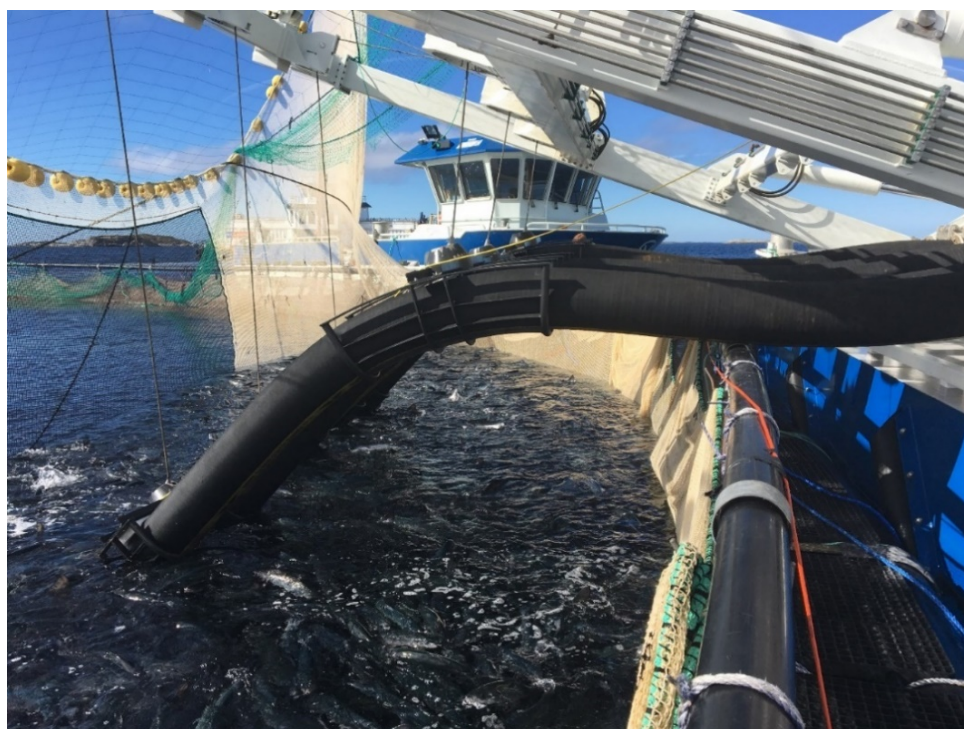
Figur 6 – Laks til avlusing pumpes fra avkast til Hydrolicer LG9332 Hydro i seks parallelle rørsystem.
