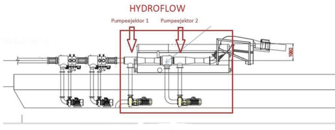
Figur 18 – Forstørret utsnitt av en linje som viser to seriekoblede enheter for lusfjerning etterfulgt av to seriekoblede Hydroflow ejektorpumper (rød boks). Utløp til silkasse (Posisjon 2) til høyre i tegningen. Kilde: Brukerhåndbok for Hydrolicer versjon 6.1, 27.4.2018
