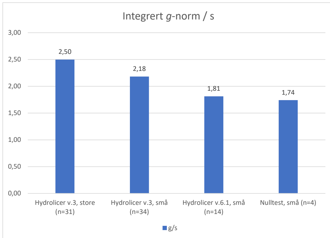
Figur 27 – Gjennomsnitt av integrert g-norm per sekund gjennomløpstid. "Nulltest" er gjennomløpstid for sensorfiskene når enhetene for avlusing ikke var innkoblede.
