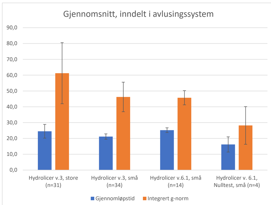
Figur 26 - Gjennomsnitt av gjennomløpstid og integrert g-norm inndelt i avlusingsystem. Data fra stor type sensorfisk i Hydrolicer versjon 6.1 er utelatt på grunn av lav N (2). "Nulltest" er gjennomløpstid for sensorfiskene når enhetene for avlusning ikke var innkoblede.
