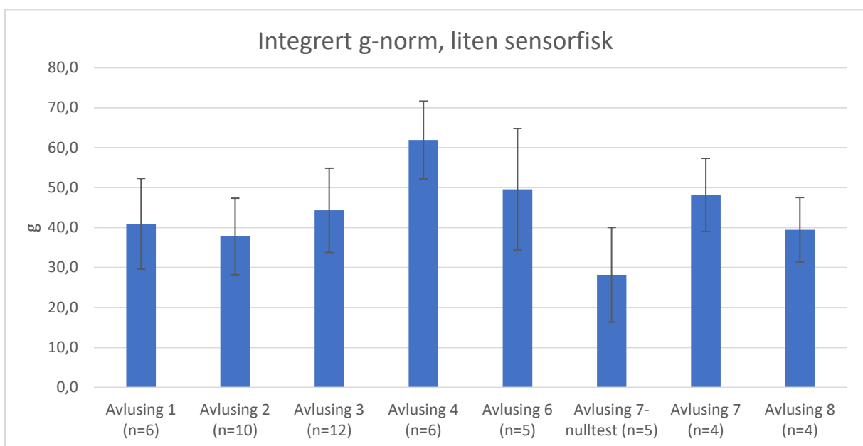
Figur 23 - Integrert g-norm for liten sensorfisk for Avlusing 1-8. Middelerverdi \pm SD. "Nulltest" er gjennomløpstid for sensorfiskene når enhetene for avlusing ikke var innkoblede.
