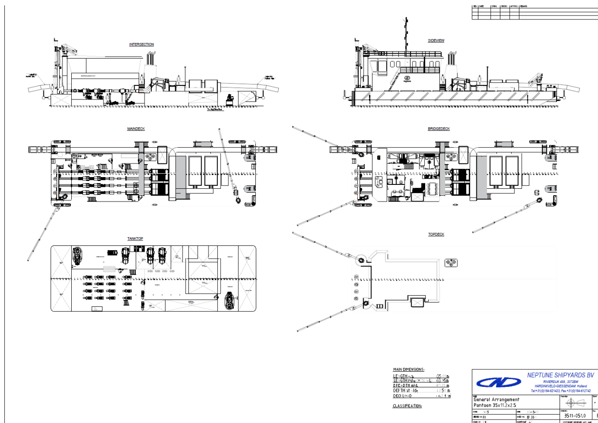
Figur 17 – Hydrolicer versjon 6.1 der fiskens innløpside er på venstre side i tegningen ovenfor. Etter avlusning kommer fisken ut i en renne med utløp til høyre eller venstre side av systemet (valgfritt). Systemet har fire linjer, hver med to lusfjerningsenheter og to ejektorpumper i serie. Kilde: MNH
