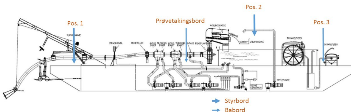
Figur 4 – Prinsippskisse for Hydrolicer LG9332 Hydro versjon 3 med seks parallelle (like) linjer. Laks i avkast pumpes inn (venstre side). Fisken passerer fisketeller, to seriekoblede enheter for lus fjerning (basert på avsuging og trykksetting av vann), en Aqua-Life Biostream BP120 fiskepumpe per linje som så løfter fisken opp til en silkasse der fisk og prosessvann separeres. Fisken går til merd i en delvis vannfylt renne og prosessvannet går til trommelfiltre som separerer ut fast stoff som lus og skjell. Figuren viser også hvor det ble tatt ut fisk til evaluering. Posisjon 1 – Fisk før avlusning ble håvet fra merd til vannfylte kar for senere prøvetaking og evaluering stress, velferd og lusetall. Posisjon 2 – Fisk
