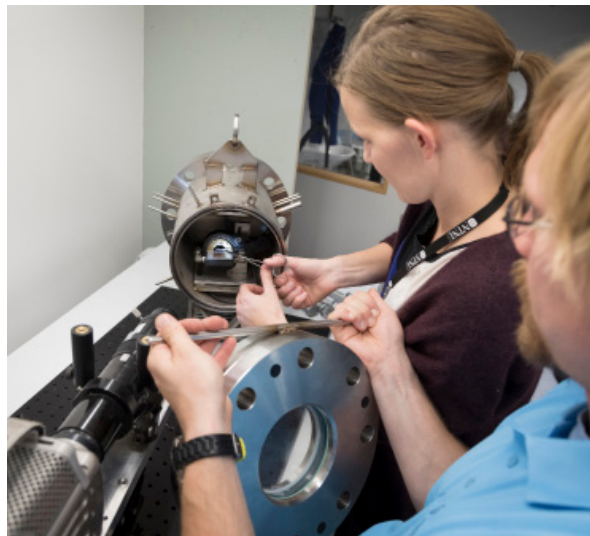
Nanostrukturert overflate plasseres inn i reaktor for å studere CO 2 -kondensasjon ved høyt trykk og lav temperatur.
