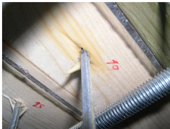
Figur 15 Fuktflekk ved håndspiker i ubehandlet trevirke
