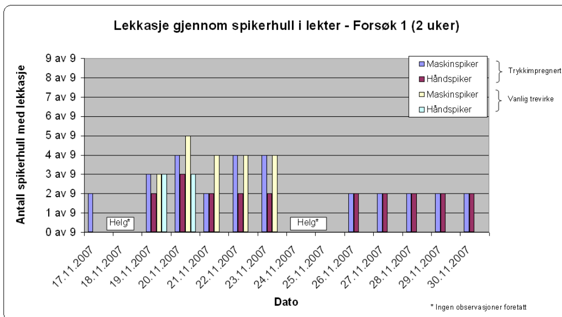
Figur 10, Lekkasje gjennom spikerhull i leker – Forsøk 1 (2 uker)
