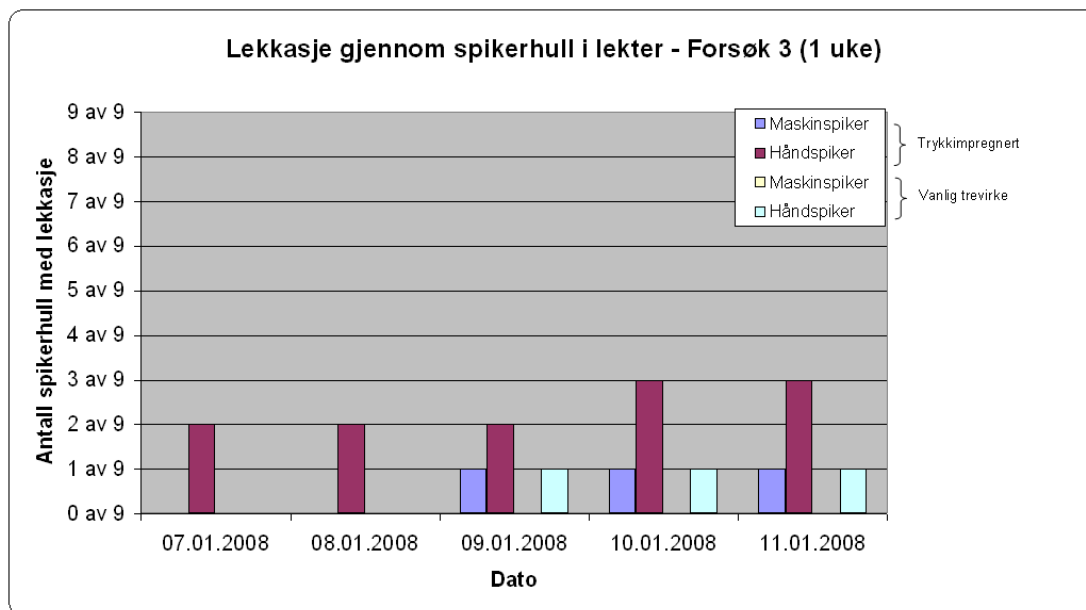
Figur 12, Lekkasje gjennom spikerhull i lekter – Forsøk 3 (1 uke)
