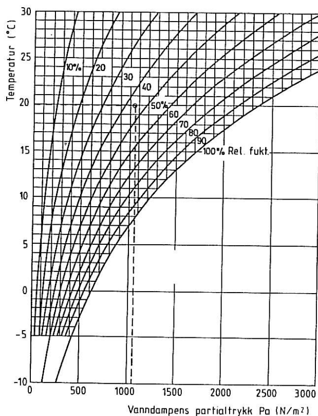
Fig. 2.1 Mollierdiagram
