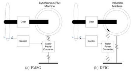
(a) PMSG
