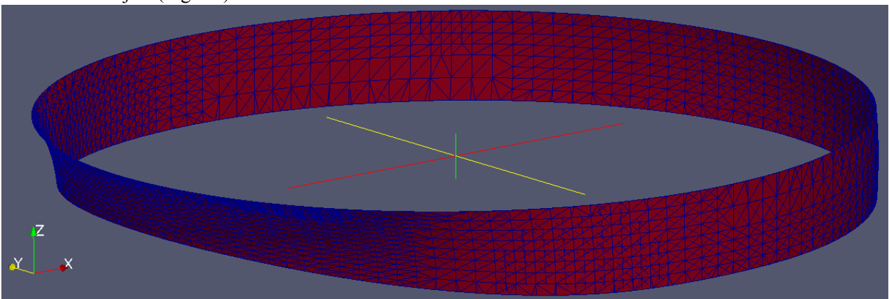
Figur 6. Deformert skjørtgeometri for simulering av strømnings i OpenFOAM.
